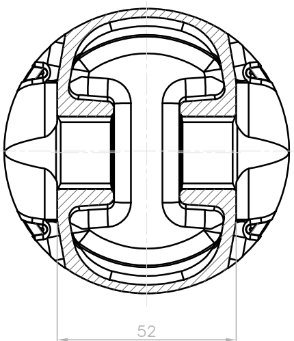
SEC:D-D
