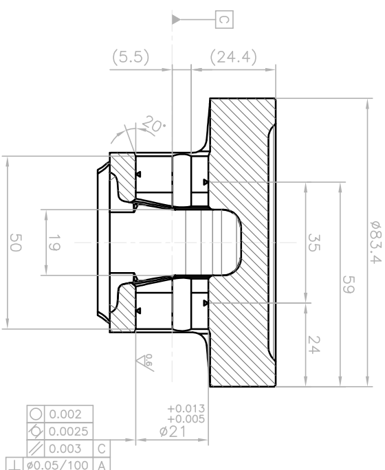
SEC:A-A
